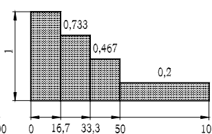
Zátěžový diagram 2
