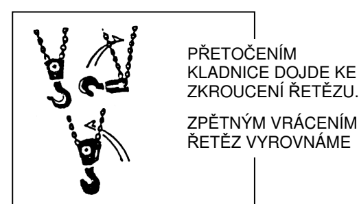
Obr. 2 Přetočení řetězu
