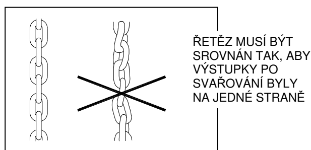
Obr. 1 Zkroucení řetězu
