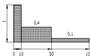
Zátěžový diagram 1
